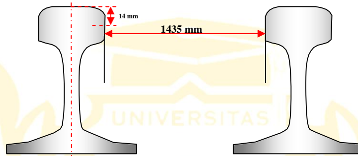
Gambar 2-2 Lebar Jalan Rel 1435 mm
