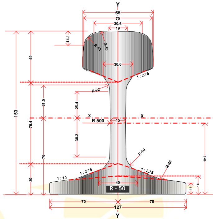
Gambar 4-2 Ukuran Penampang Rel R.50
