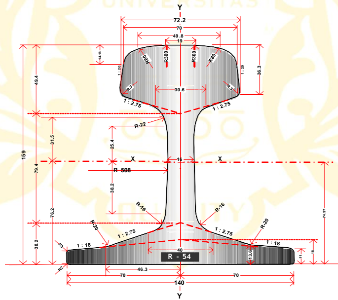
Gambar 4-3 Ukuran Penampang Rel R.54
