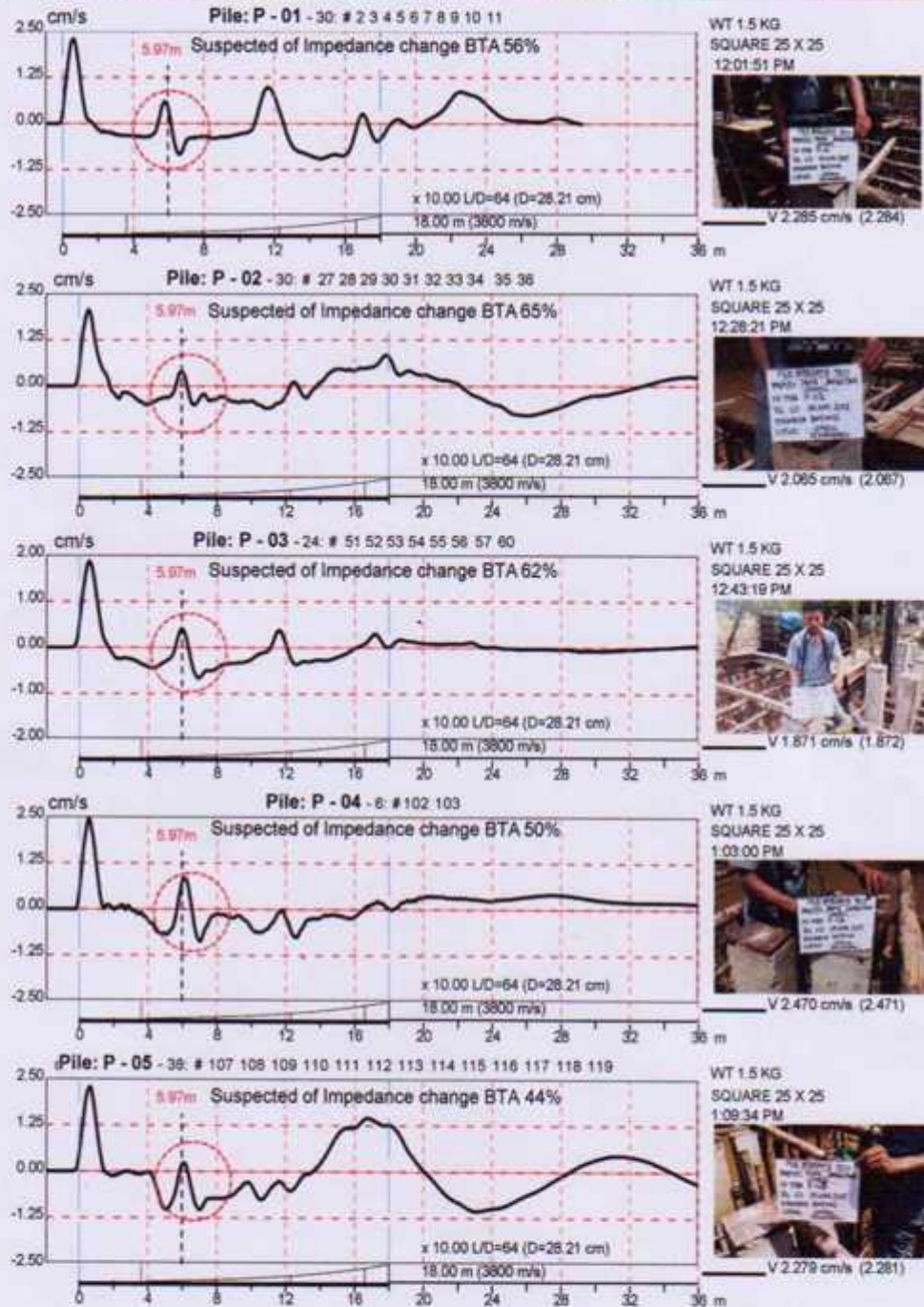
Gambar 4.2 Hasil Analisa Rambatan Gelombang Pada Penelitian Tiang Pondasi
